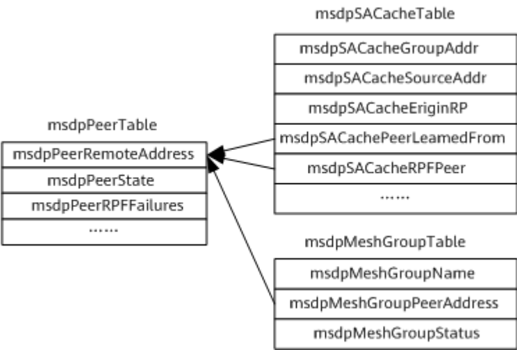
图 163-1 msdpPeerTable 与 msdpSACacheTable、msdpMeshGroupTable 关系图
